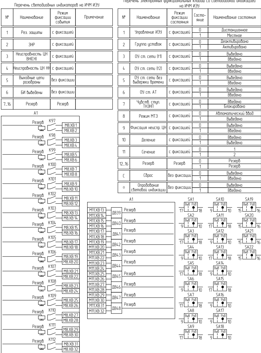
Рисунок В.6 – Схема электрическая принципиальная (часть 6)
